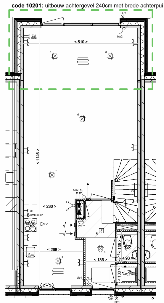
begane grond
