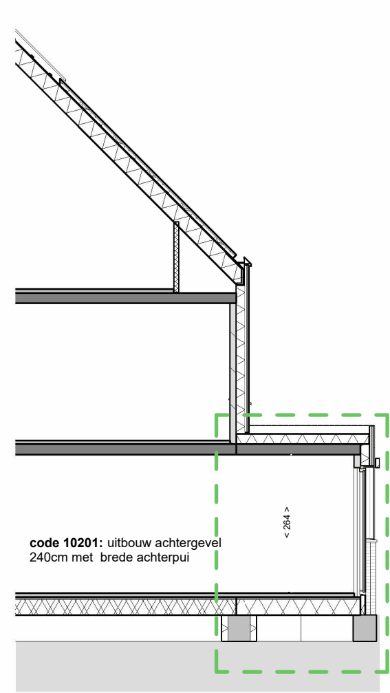
doorsnede
