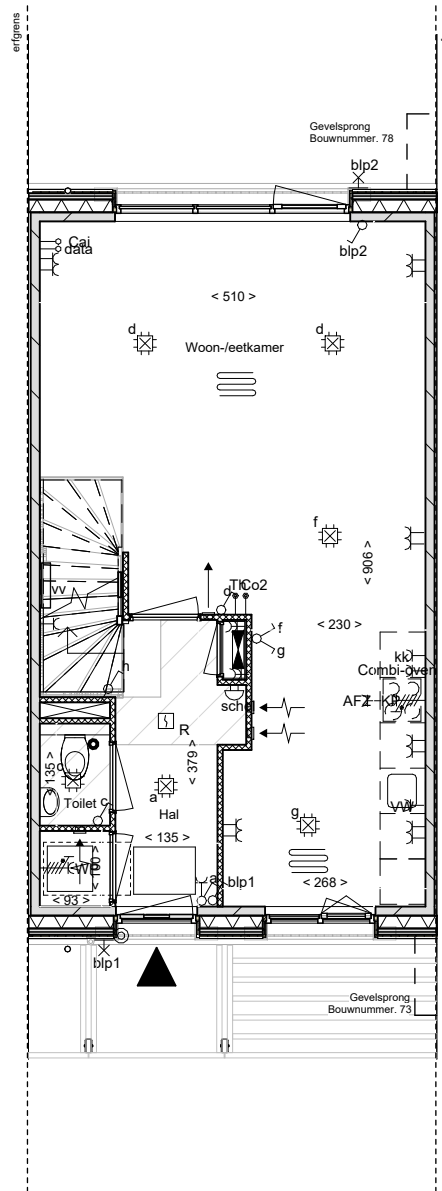
begane grond
